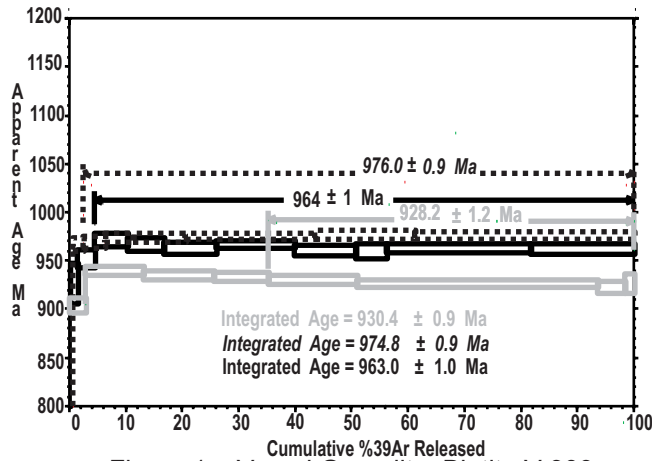
Figure 1e. Vergel Granulite, Biotite V-309
